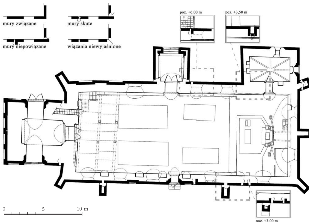
Ilustracja 2. Mołtajny, kościół parafialny, rzut z oznaczeniem węzłów badawczych; oprac. autorzy
