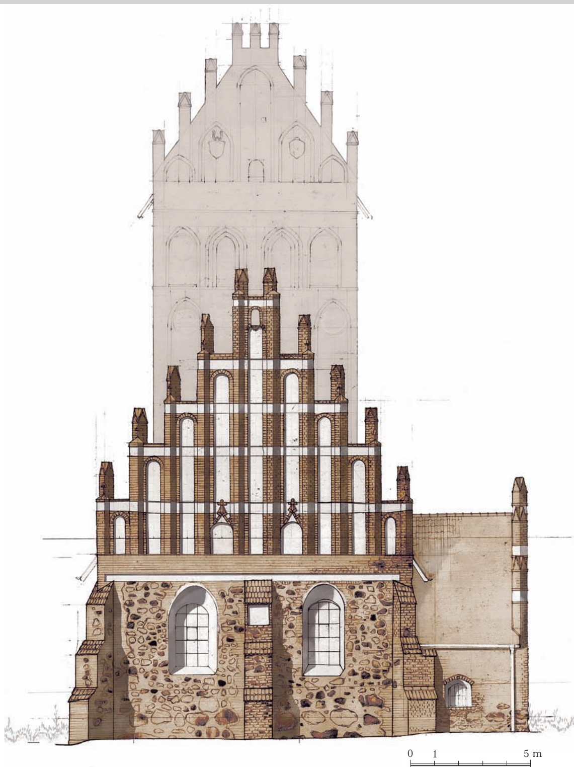
Ilustracja 1. Mołtajny, kościół parafialny, elewacja wschodnia, inwentaryzacja; rys. Katarzyna Wysocka, Maria Wolska
