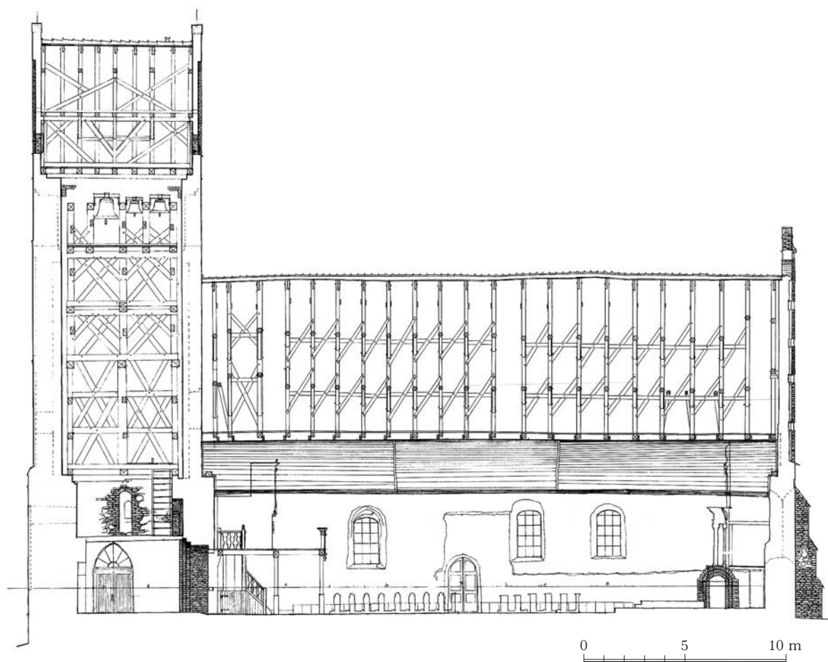
Ilustracja 5. Mołtajny, kościół parafialny, przekrój podłużny; rys. Marek Patrzałek, Stanisław Podsiadło, Olga Zawistowska
