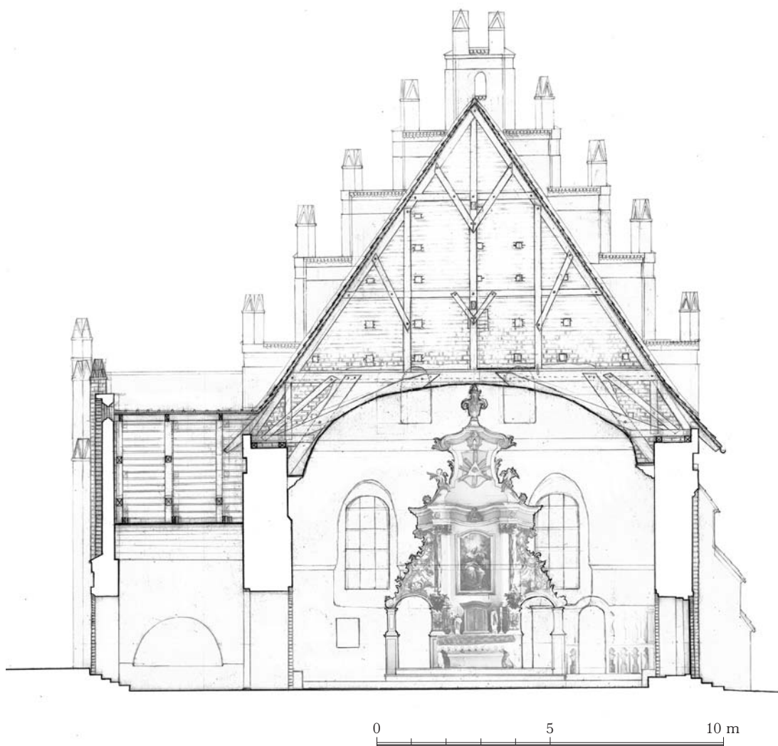
Ilustracja 6. Mołtajny, kościół parafialny, przekrój poprzeczny; rys. Julia Lipska, Emilia Oniszczyk
