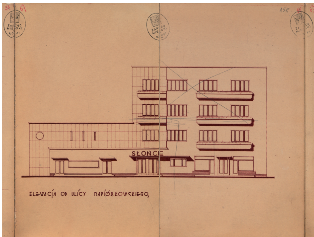
Ilustracja 15. I. Fajnberg, projekt kinoteatru przy ul. Przybyszewskiego 16 w Łodzi, APŁ, zesp. Urząd Dzielnicowy Łódź-Górna, sygn. 17342
